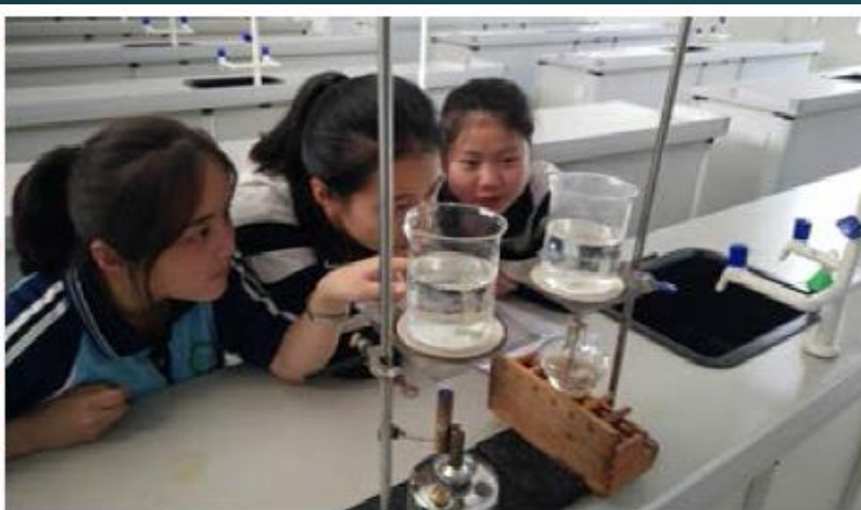
模拟大气对流运动
